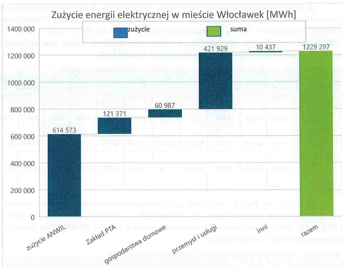
Rys. 21 Zużycie energii elektrycznej w mieście Włocławek w 2023 r.
