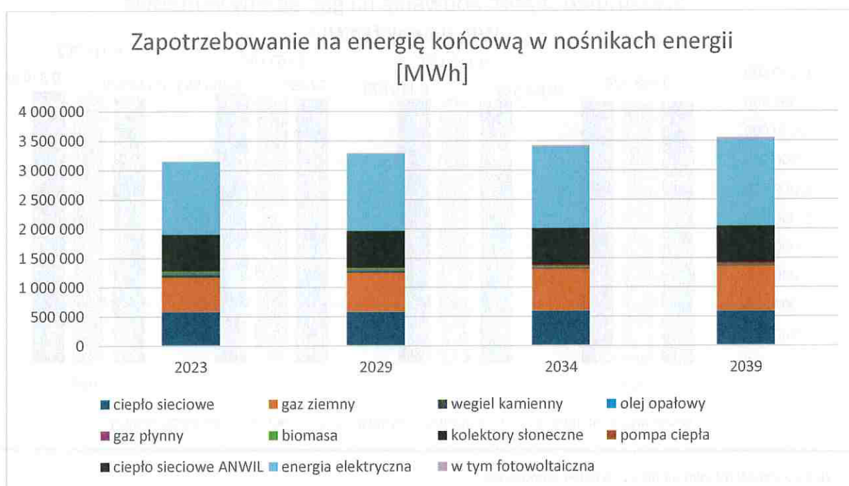
Rys. 28 Zapotrzebowanie na energię końcową w nośnikach energii – prognoza
