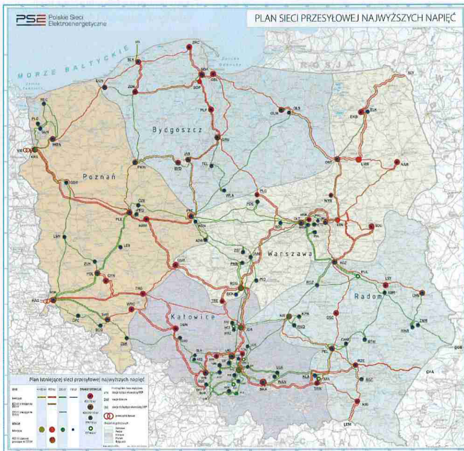
Rys. 12 Schemat Krajowego Systemu Przesyłowego (KSE)
