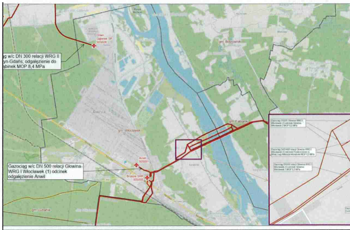
Rys. 17 Schemat sieci przesyłowej gazu ziemnego na terenie miasta Włocławek
