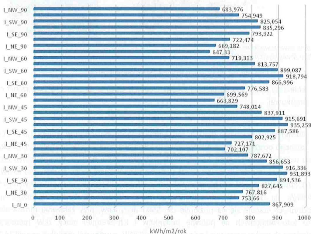
Rys. 5 Wartość promieniowania słonecznego na jednostkę powierzchni
