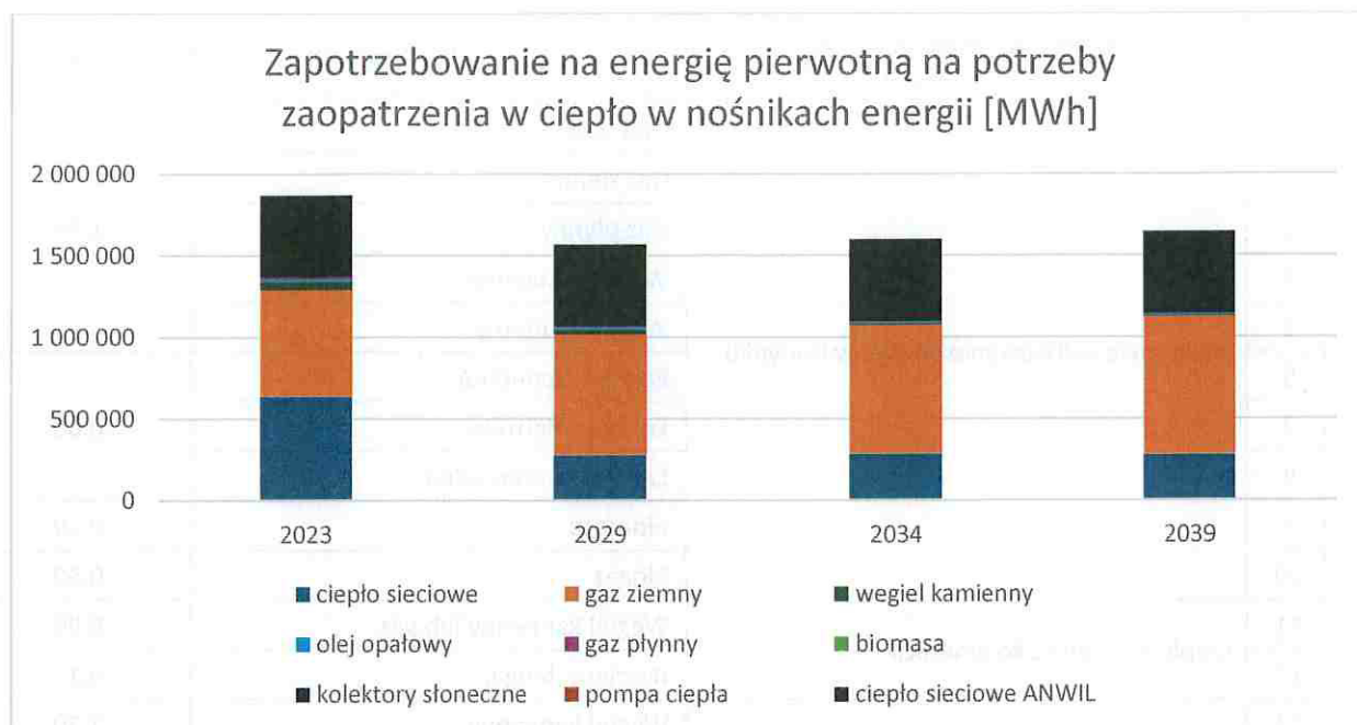
Rys. 29 Zapotrzebowanie na energię pierwotną na potrzeby zaopatrzenia w ciepło – perspektywy Źródło: Opracowanie własne
