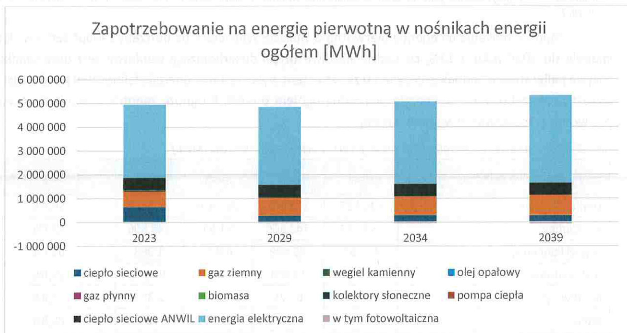
Rys. 30 Zapotrzebowanie na energię pierwotną ogółem – perspektywy Źródło: Opracowanie własne
