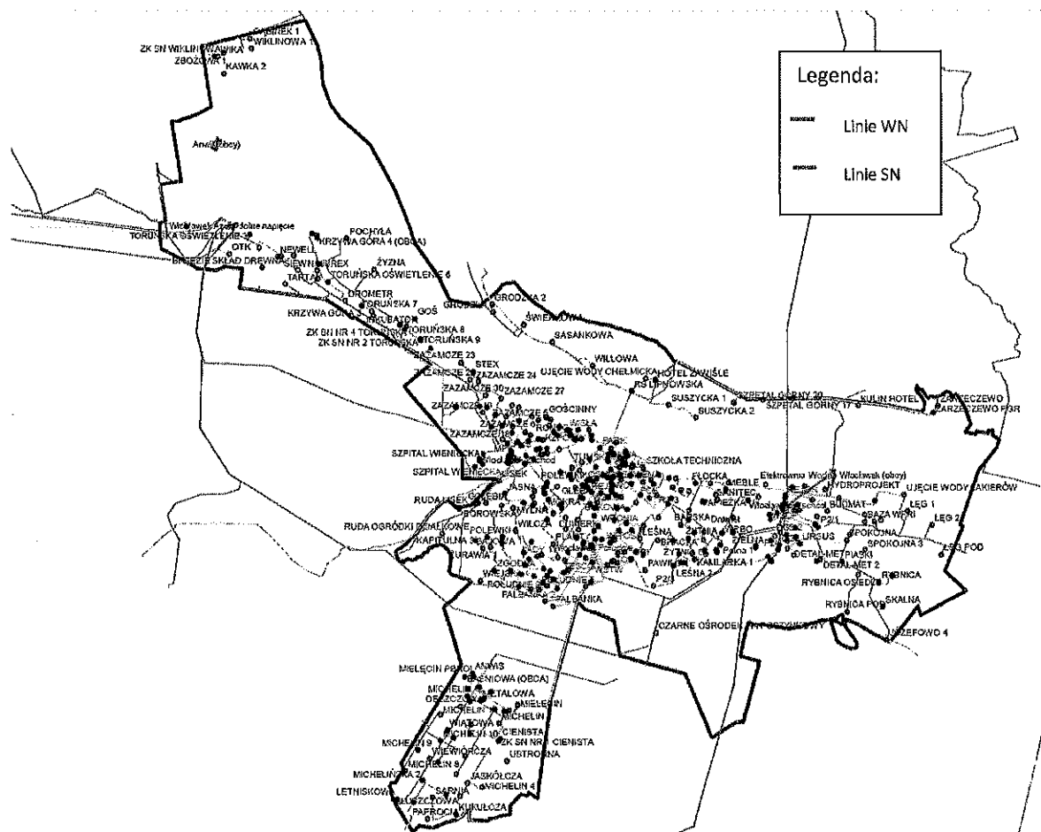
Rys. 14 Schemat sieci elektroenergetycznej SN na terenie miasta Włocławek. Źródło: ENERGA Operator S.A.
