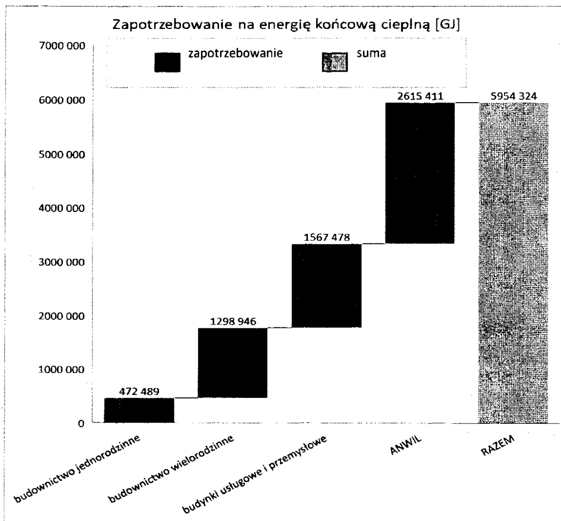
Rys. 16 Zapotrzebowanie na energię końcową cieplną w mieście Włocławek Źródło: Opracowanie własne
