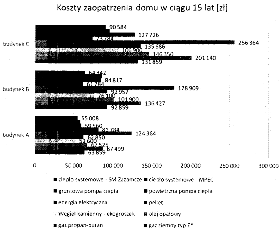
Rys. 7 Analiza kosztów zaopatrzenia domu w ciepło przez okres 15 lat (w cenach stałych)
