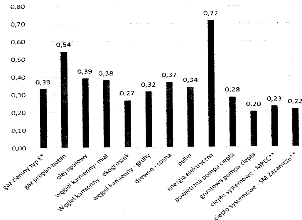
Rys. 6 Porównanie kosztów produkcji ciepła (brutto)
