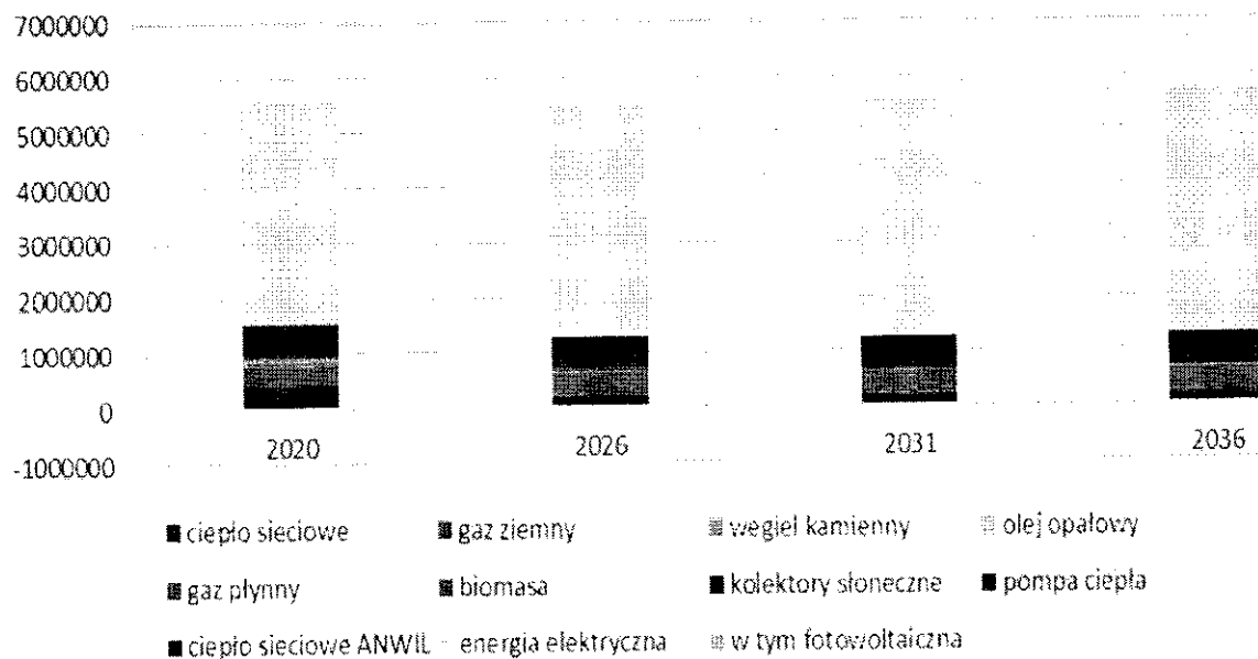
Rys. 26 Zapotrzebowanie na energię pierwotną – perspektywy
