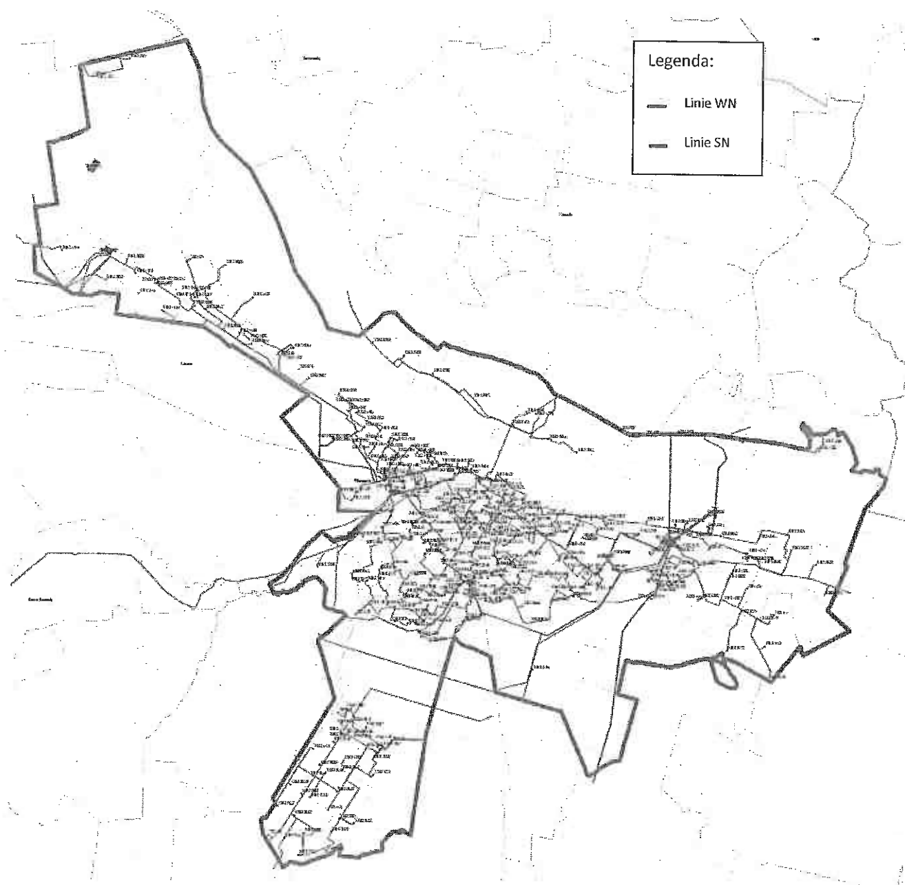
Rys. 11 Schemat sieci elektroenergetycznej SN na terenie miasta Włocławek.
